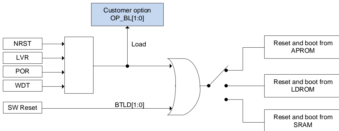
SC32F12T/12G 复位后启动区域切换示意图
