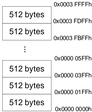
SC32F12xx8 系列 256 Kbytes APROM Sector 分区示意
