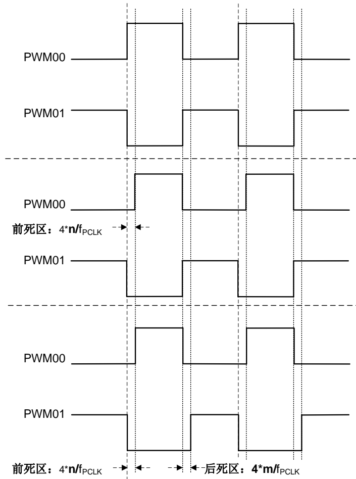
PWM0 死区输出波形
