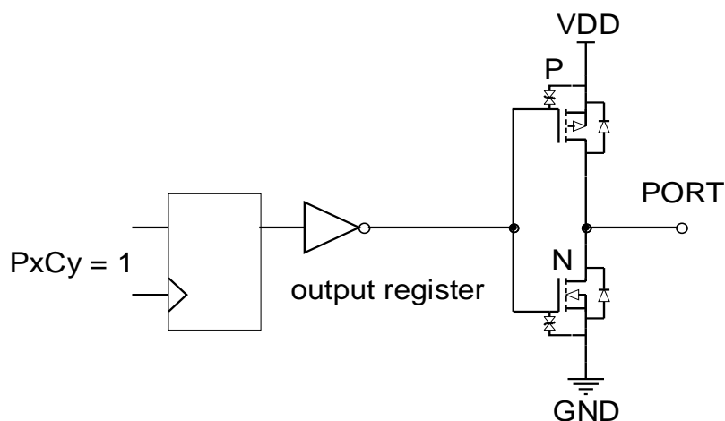
强推挽输出模式的端口结构示意图
