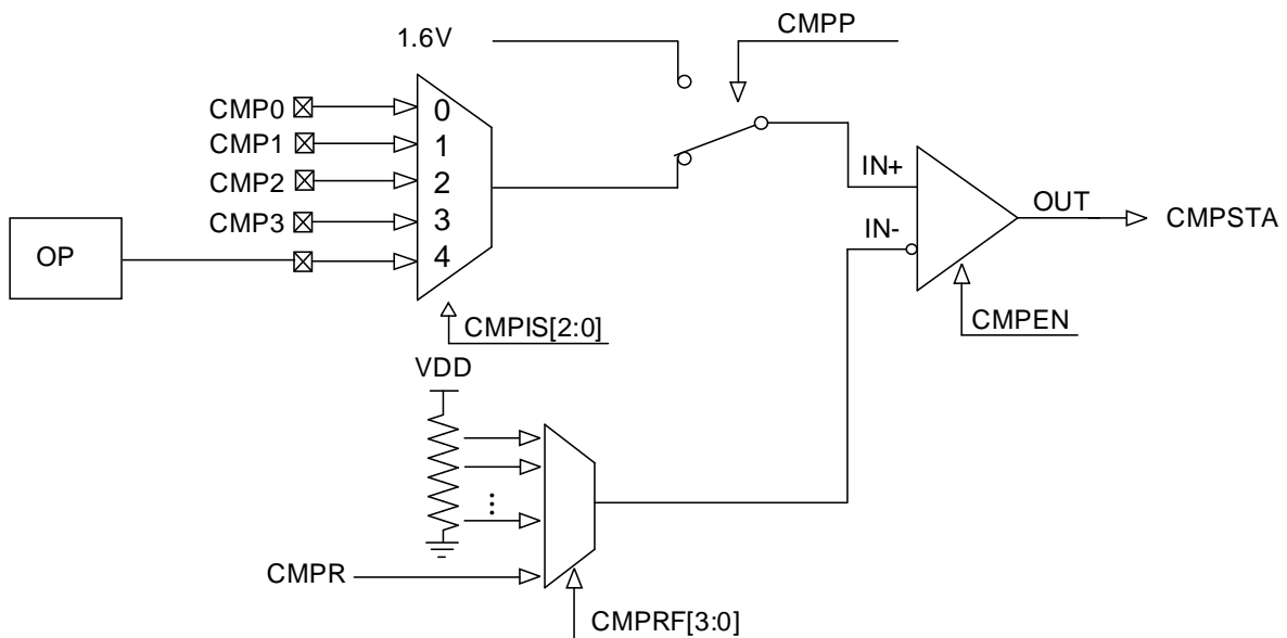
模拟比较器结构框图
